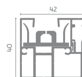
Guida zip laterale
