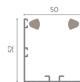
Profilo compensatore
