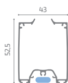
Cassonetto
