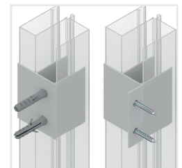
Staffe di fissaggio a scomparsa cod. 382-398
