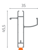
Barramaniglia
